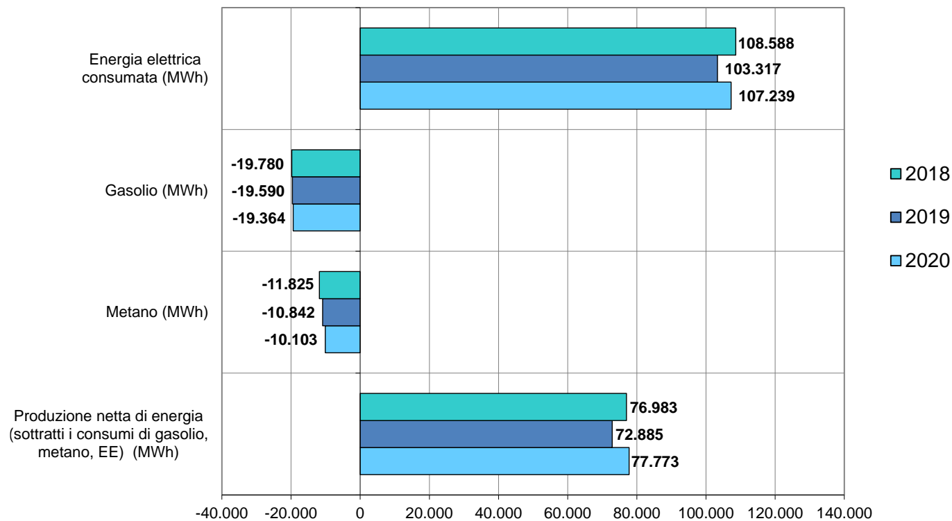
Figura 8: Bilancio energetico
