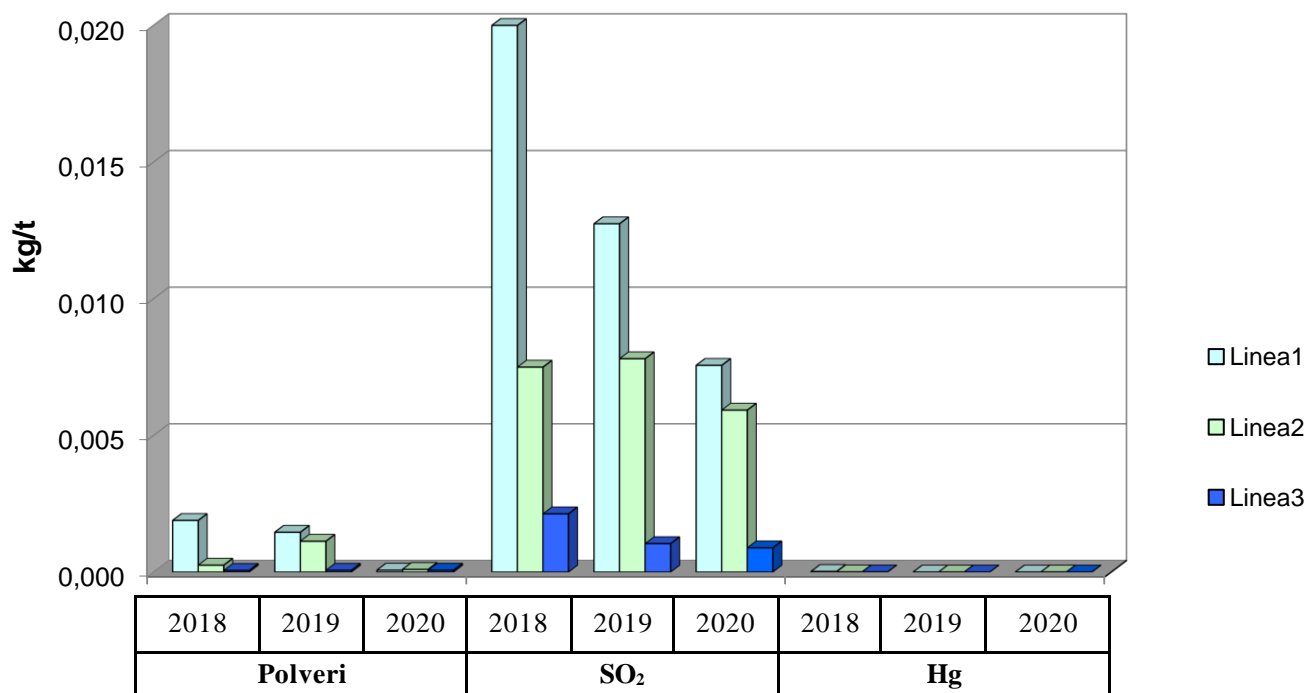
Figura 22: Andamento dell'indicatore "Fattori di Emissione(Polveri, SO 2 , Hg)"
