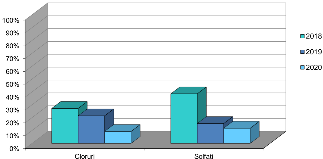
Figura 12: Andamento dell'indicatore "Posizionamento Rispetto al Limite" (S1) (Cloruri, Solfati)
