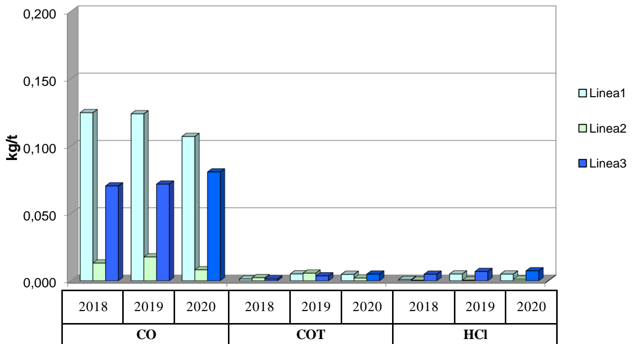
Figura 21: Andamento dell'indicatore "Fattori di Emissione(CO, COT, HCl)"
