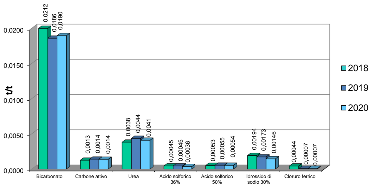
Figura 25: Andamento dell'indicatore "Fattore di utilizzo reagenti"
